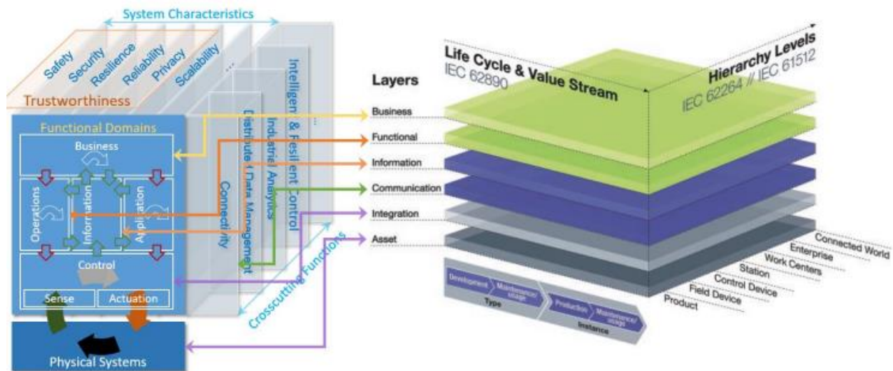
図表 9: IIRA (左) と RAMI (右) の機能マッピング
