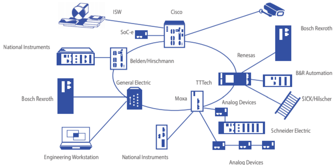
図表 15: 複数のベンダー機器で構成される TSN テストベッドの設計概要
