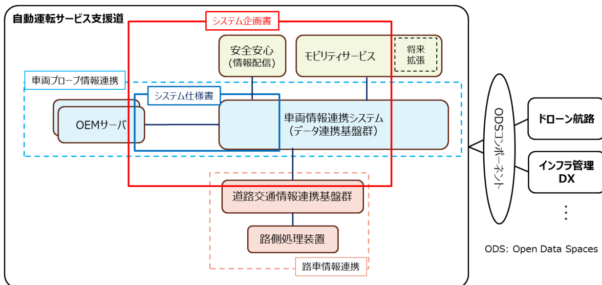
図 3：DADC が想定する自動運転サービス支援道の社会システムおよび検討スコープのイメージ
