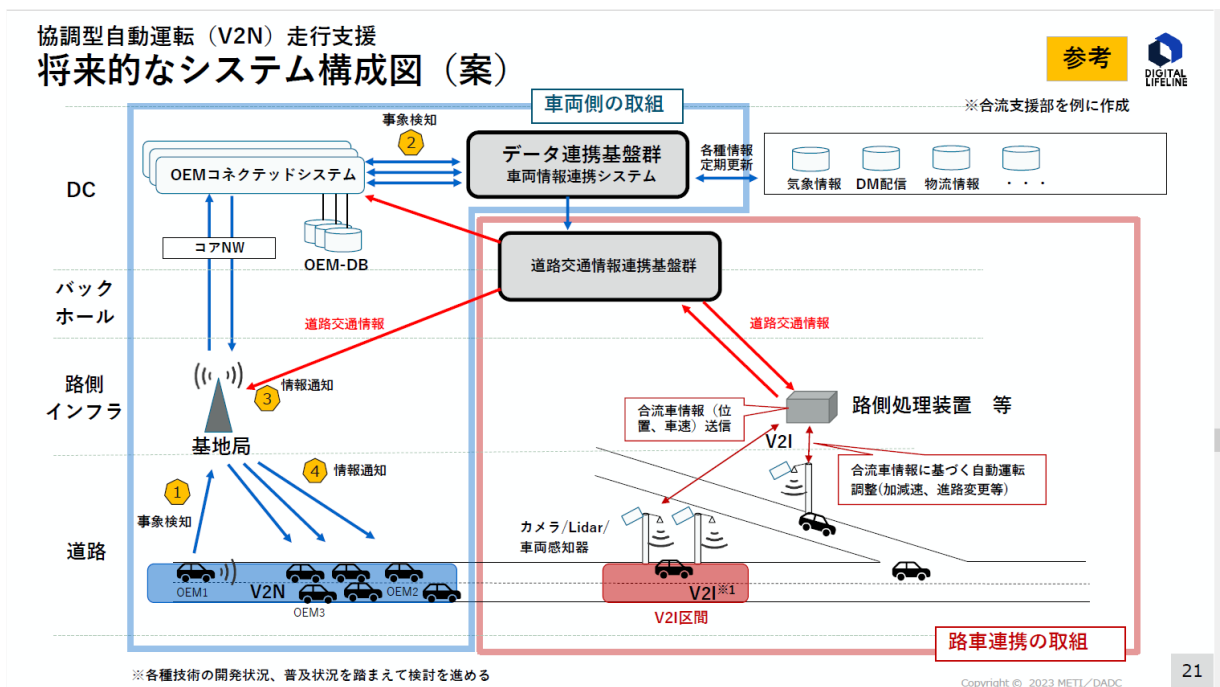
図1：第2期第1回自動運転サービス支援道普及戦略WGで提示した将来的なシステム構成図（案）
