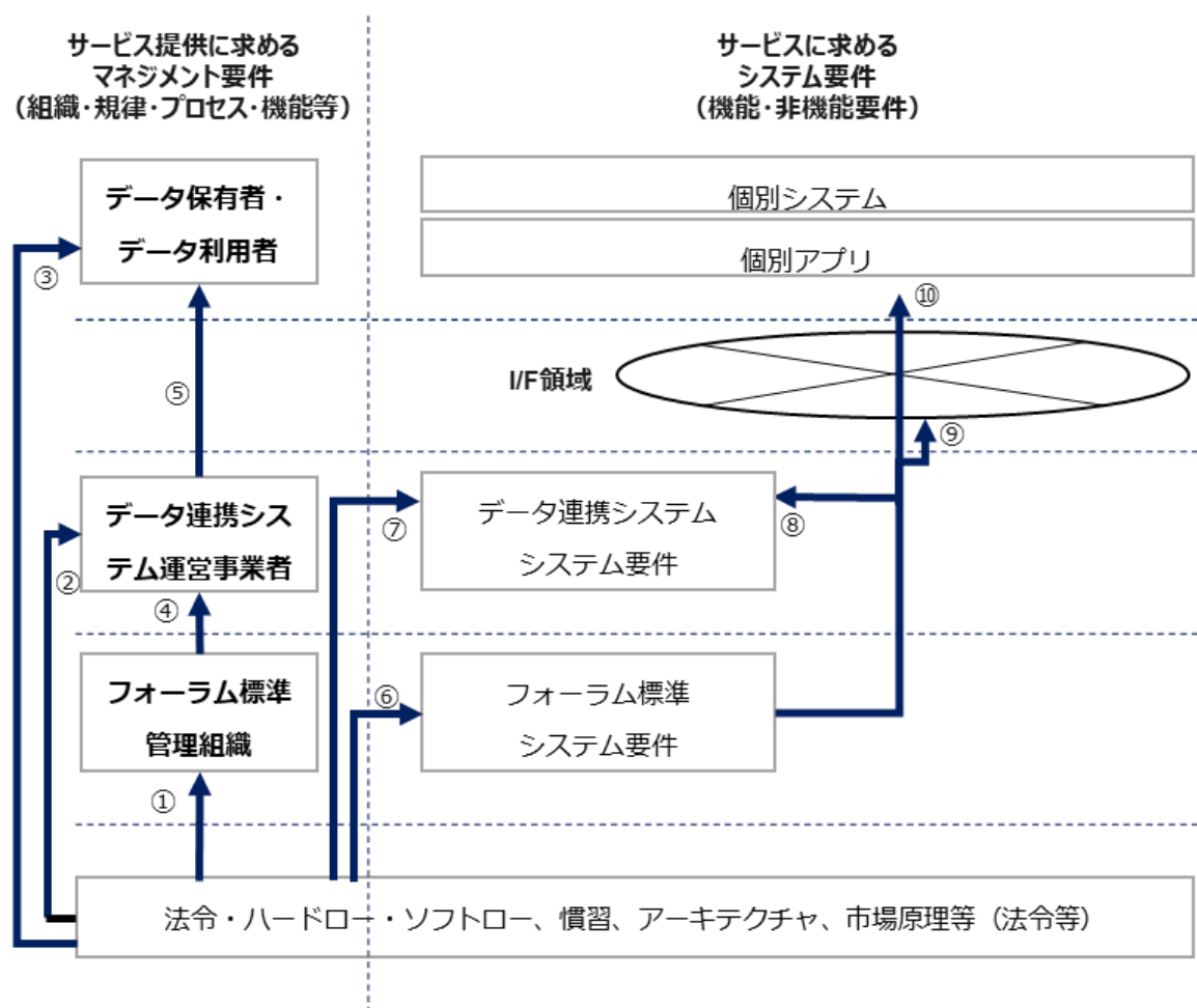
図 1 フォーラム標準に関するガバナンスの分類
