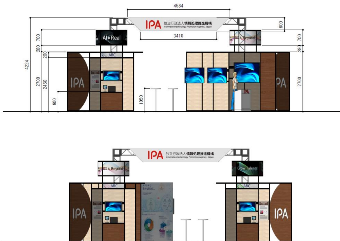
図2 立面図
