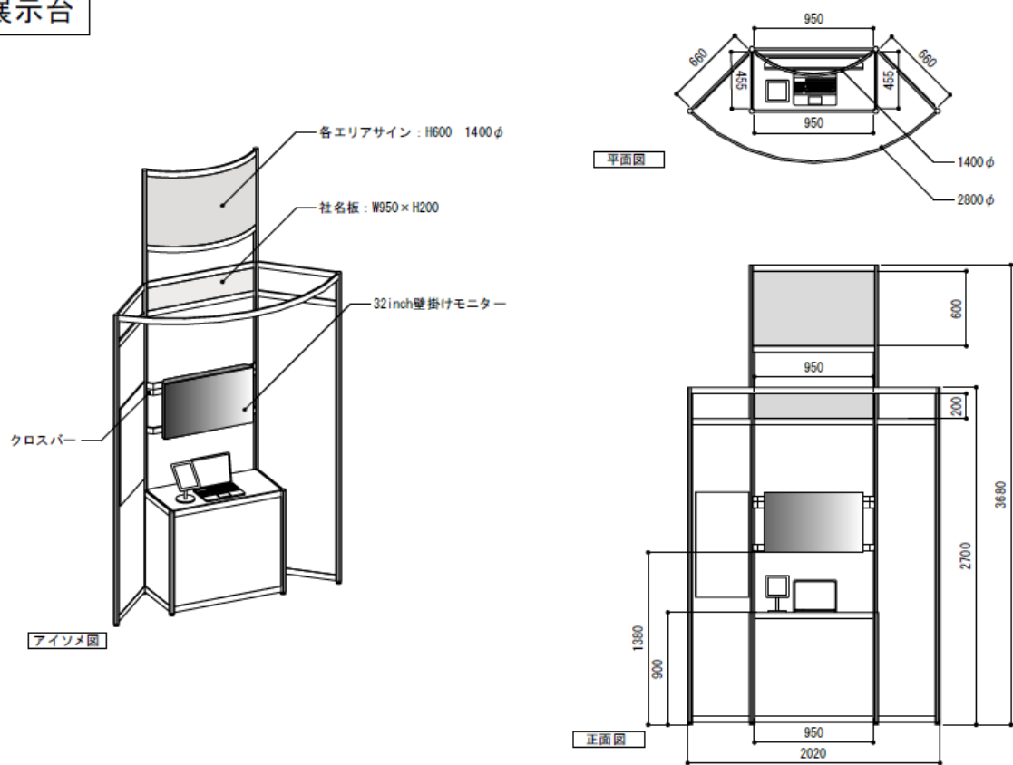
図5 展示台図
