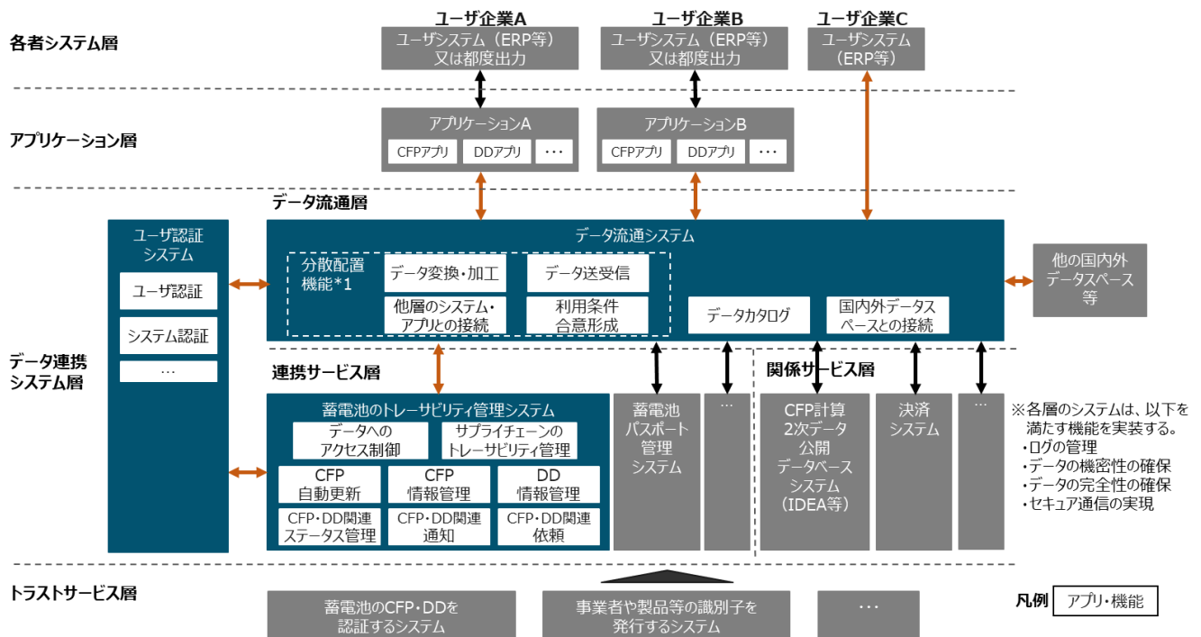
図1 データ連携基盤のシステムアーキテクチャ
