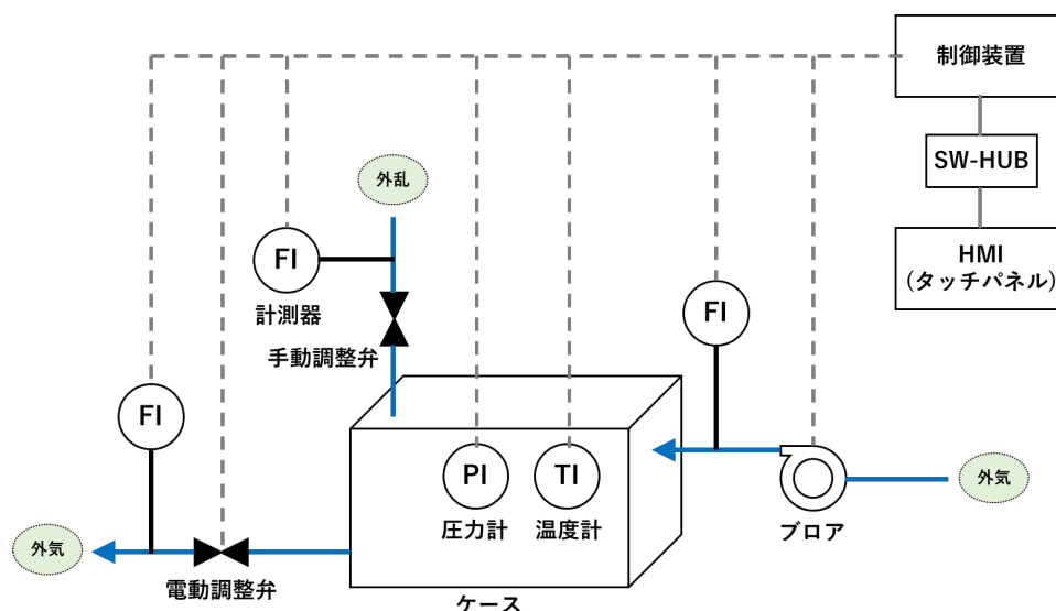
図1 可搬型演習用模擬プラントのシステム構成例
