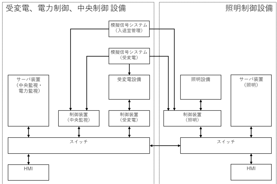
図1 可搬型演習用模擬プラントのシステム構成例
