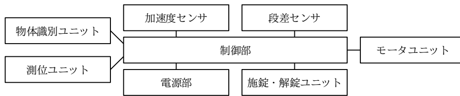
図2 スーツケースのシステム構成
