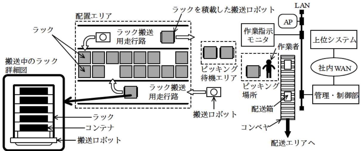
図1 従来の自動倉庫システムの例
