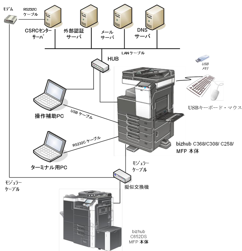
図7-1 開発者テストの構成図
