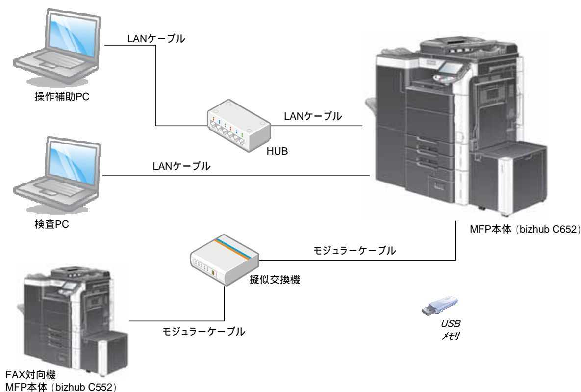
図3-2 侵入テストの構成図
