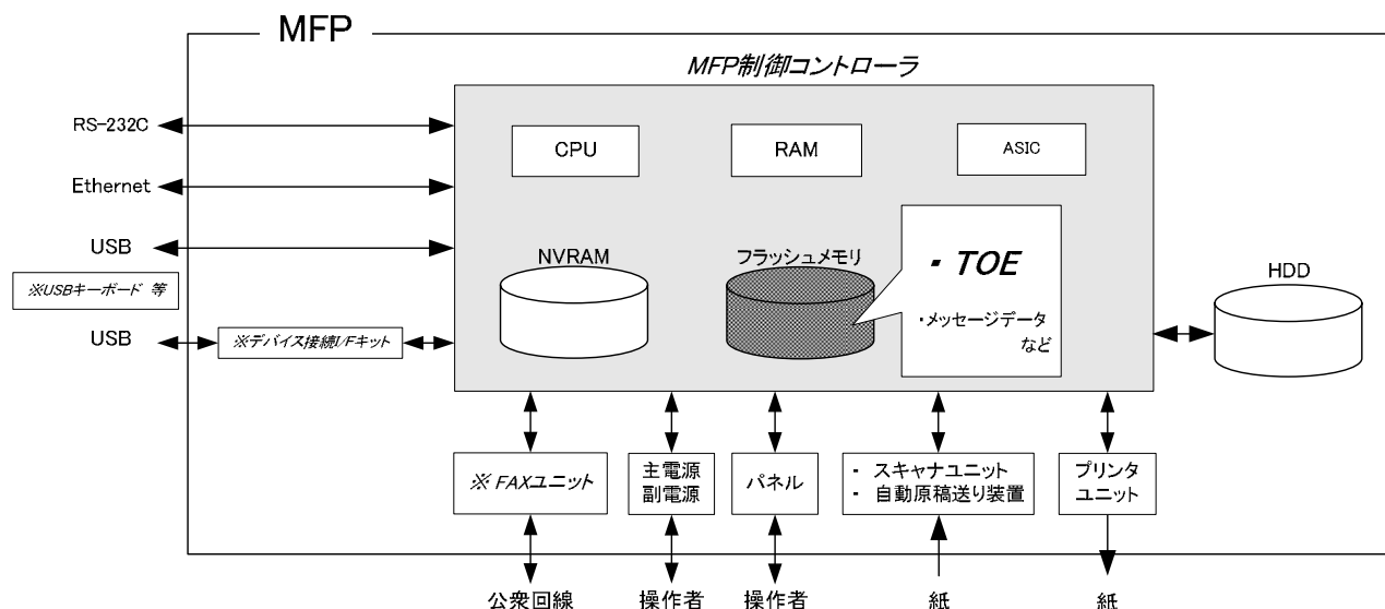
図1-1 TOEに関するハードウェア構成
