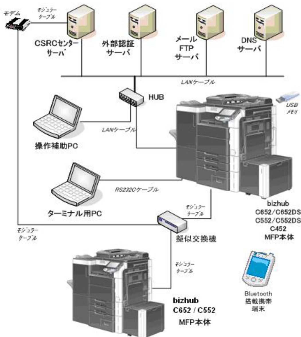
図3-1 開発者テストの構成図
