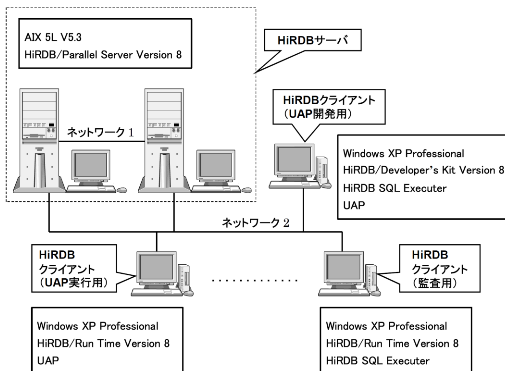
図1-3 TOEの動作構成
