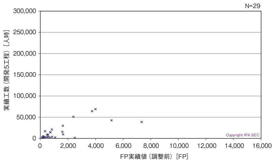
図表 6-3-9 ● FP 規模と工数（新規開発、IFPUG グループ）
