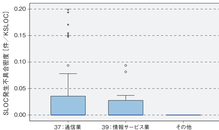
図表 9-3-11 ● 業種（中分類）別 SLOC 発生不具合密度（改良開発） 箱ひげ図
