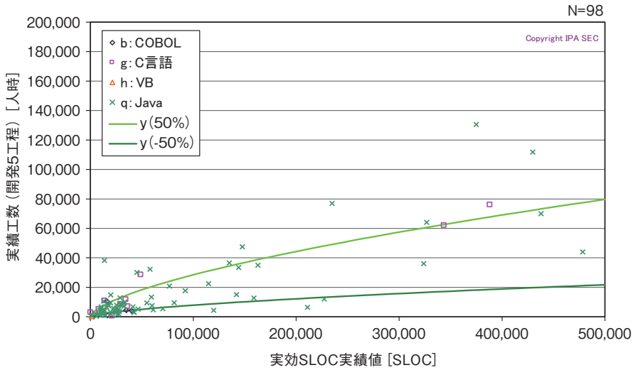
図表 6-4-7 ● 主開発言語別の SLOC 規模と工数（新規開発） 拡大図（信頼区間 50% 付き）（SLOC 規模 \leq 500,000 & 工数 \leq 200,000 ）
