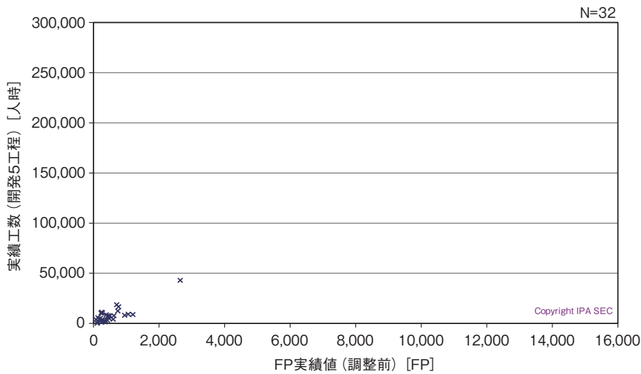
図表 6-3-14 ● FP 規模と工数（改良開発、FP 計測手法混在）
