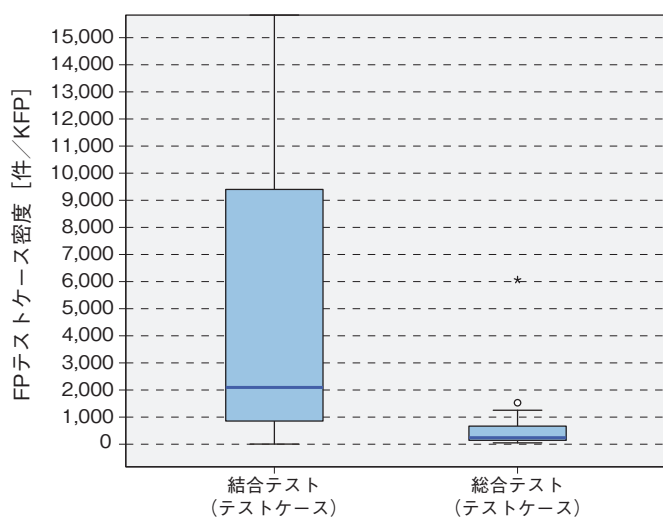
図表 7-5-6 ● FP 規模あたりのテストケース数 (新規開発、IFPUG グループ) 箱ひげ図
