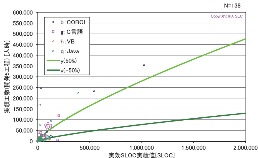
図表 6-4-15 ● 主開発言語別の SLOC 規模と工数（改良開発）（信頼区間 50% 付き）
