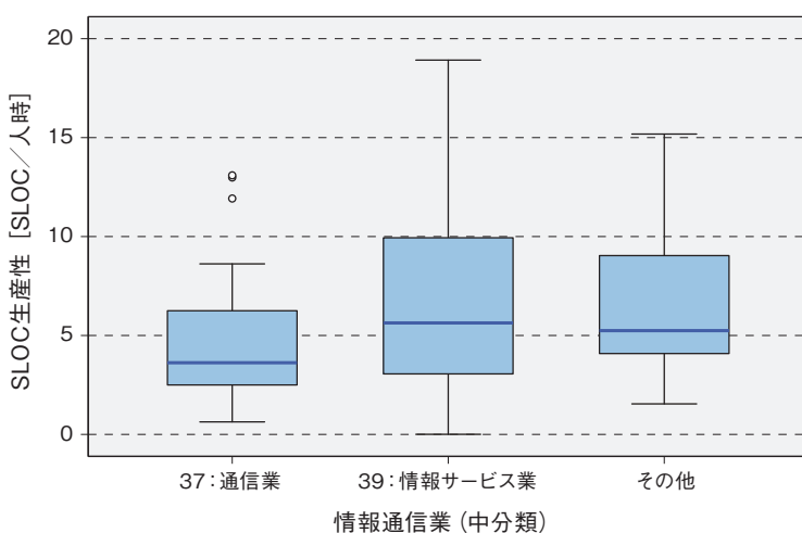
図表 8-3-18 ● 業種別（中分類）SLOC 生産性（新規開発）箱ひげ図
