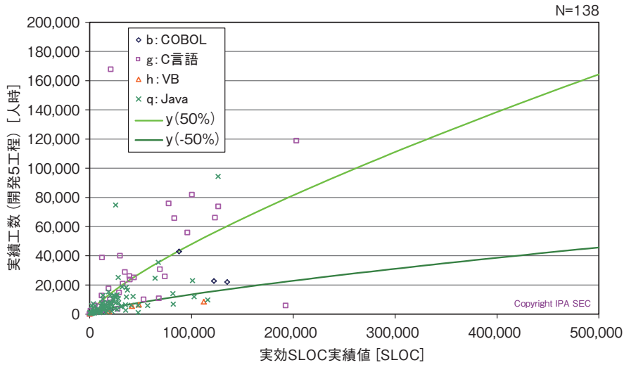
図表 6-4-16 ● 主開発言語別の SLOC 規模と工数 (改良開発) (信頼区間 50% 付き) 拡大図 (SLOC 規模 ≤ 500,000 & 工数 ≤ 200,000)
