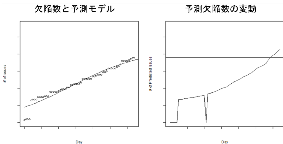
図 3-4-21 2017P7 の欠陥数と信頼性モデルと予測欠陥数の変動
