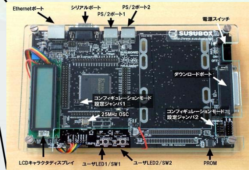
開発したFPGAボード
