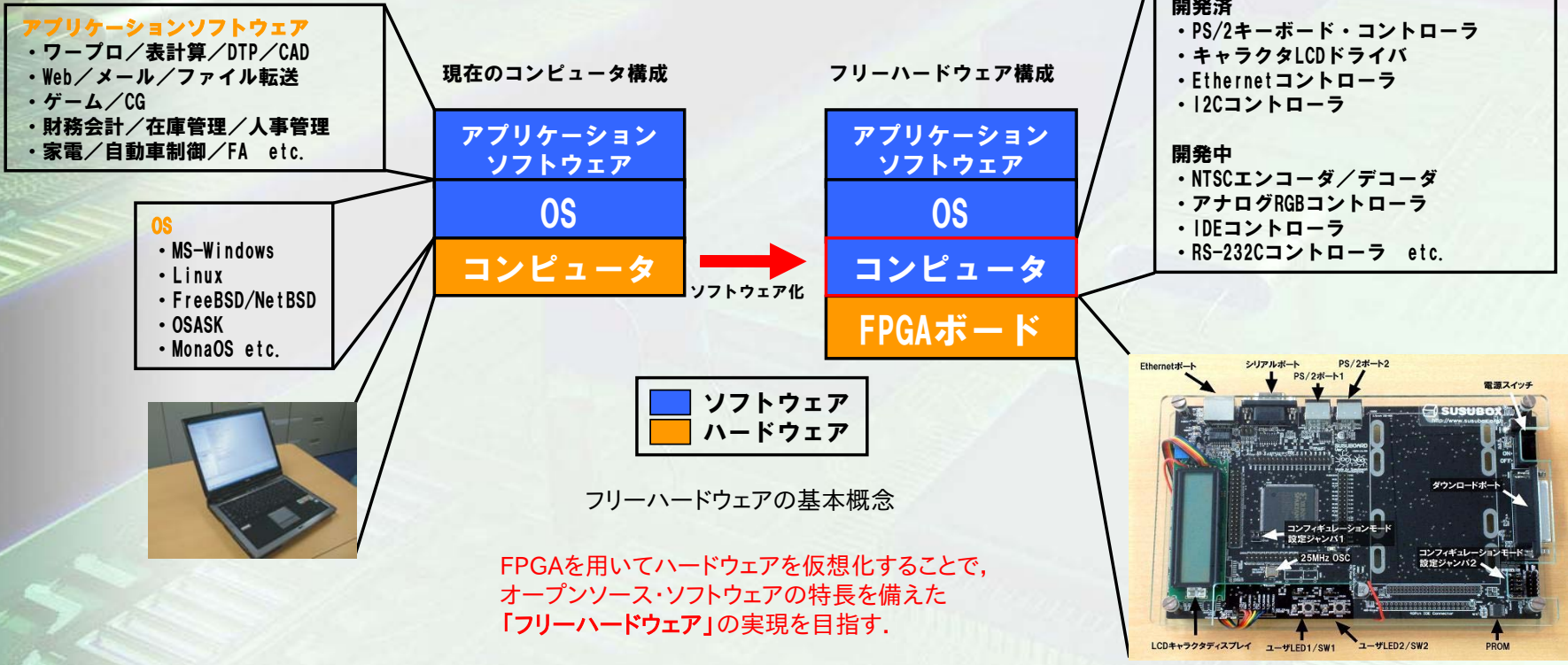
開発したFPGAボード
