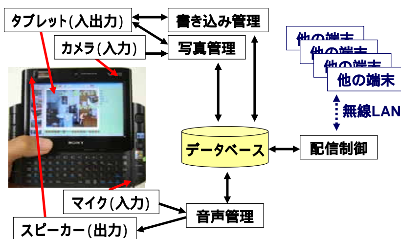
図 1 PhotoChat のシステム構成
