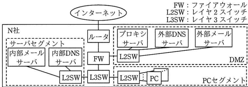
図1 N社の情報システムの構成
