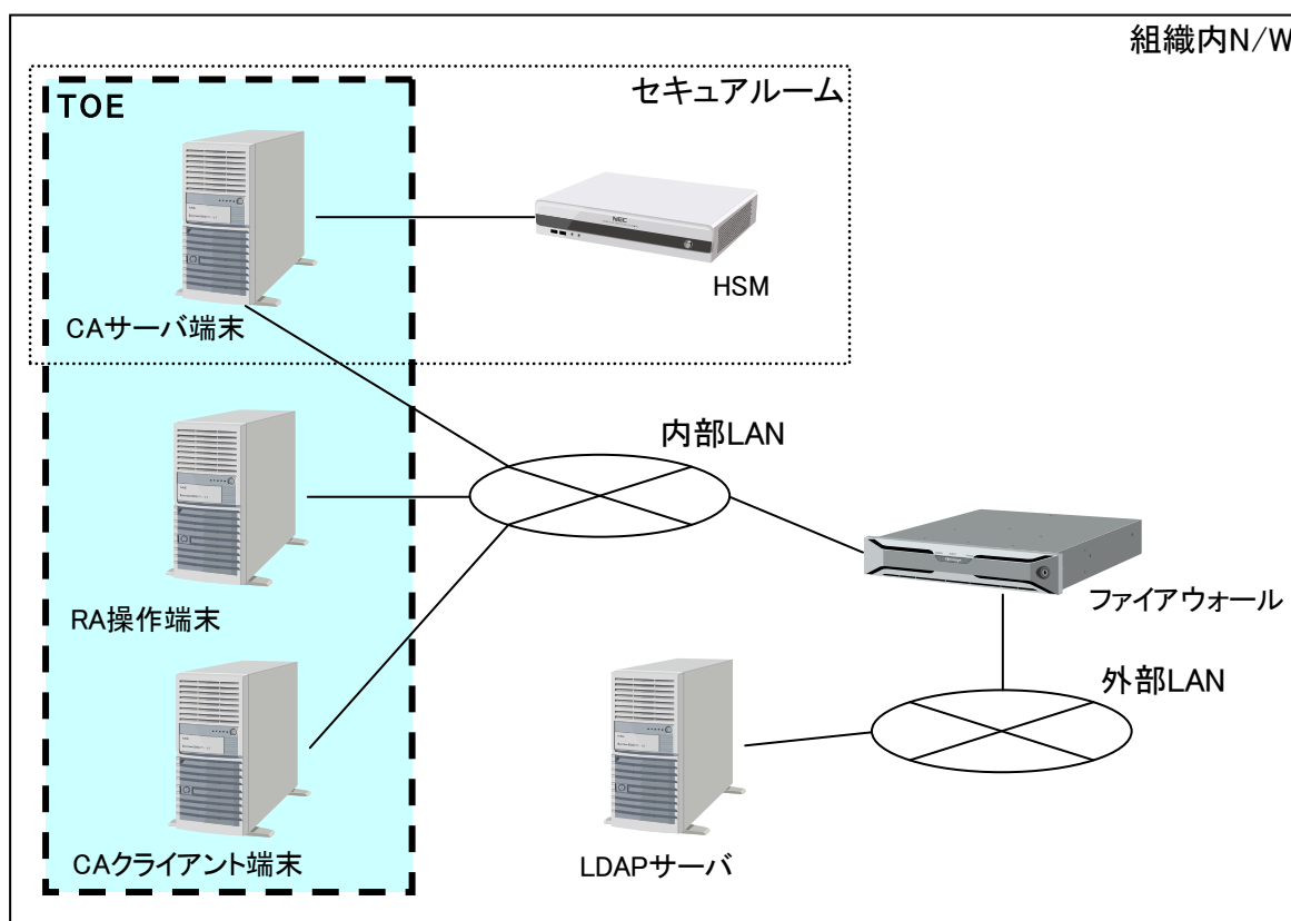
図1-1 PKIサーバ/Carassuit 電子政府版 ver6.0のIT構成図
