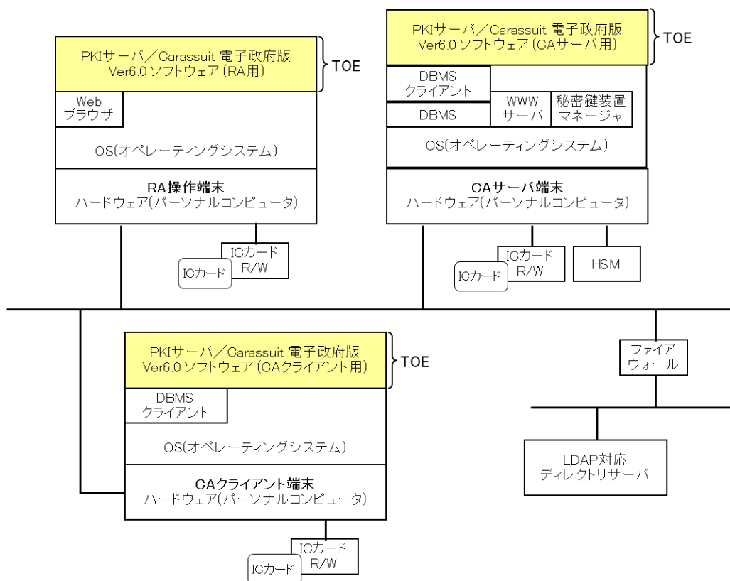
図1-2 PKIサーバ/Carassuit 電子政府版 ver6.0の構成図
