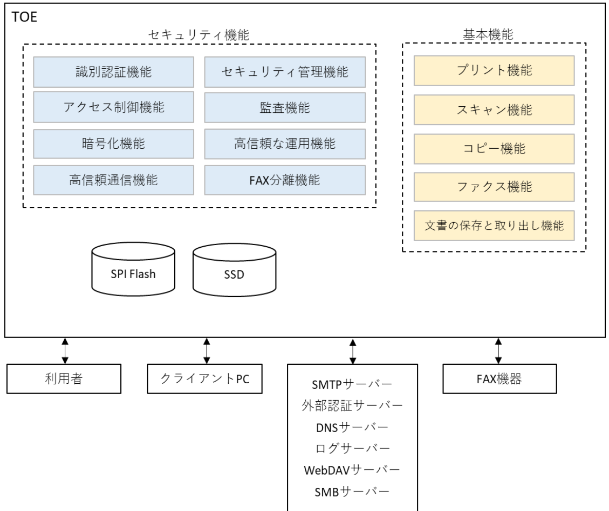
図 5-1 TOE の構成
