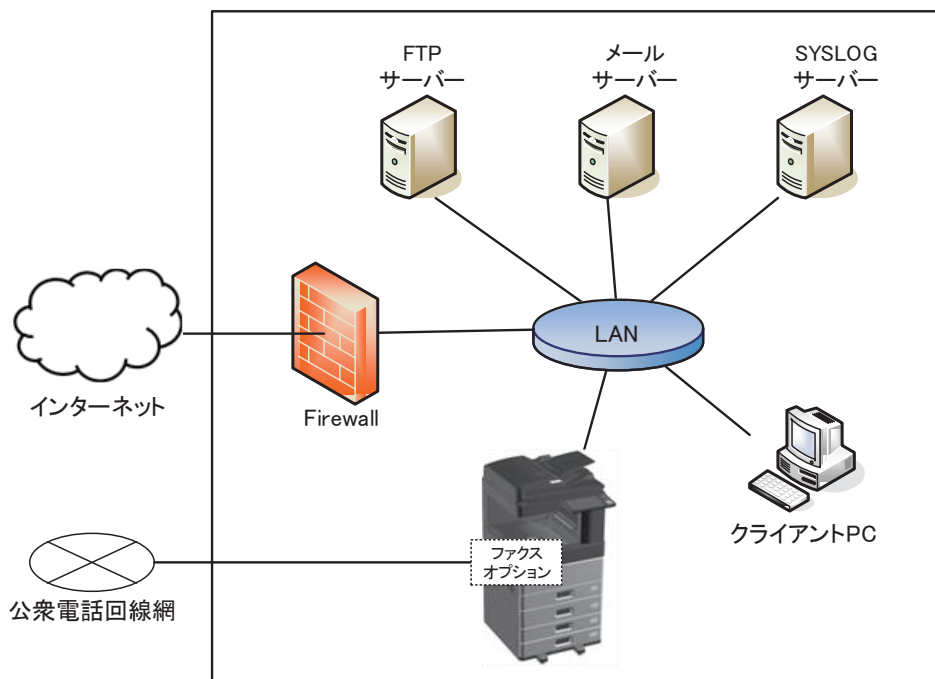
図 1 MFP の利用環境
