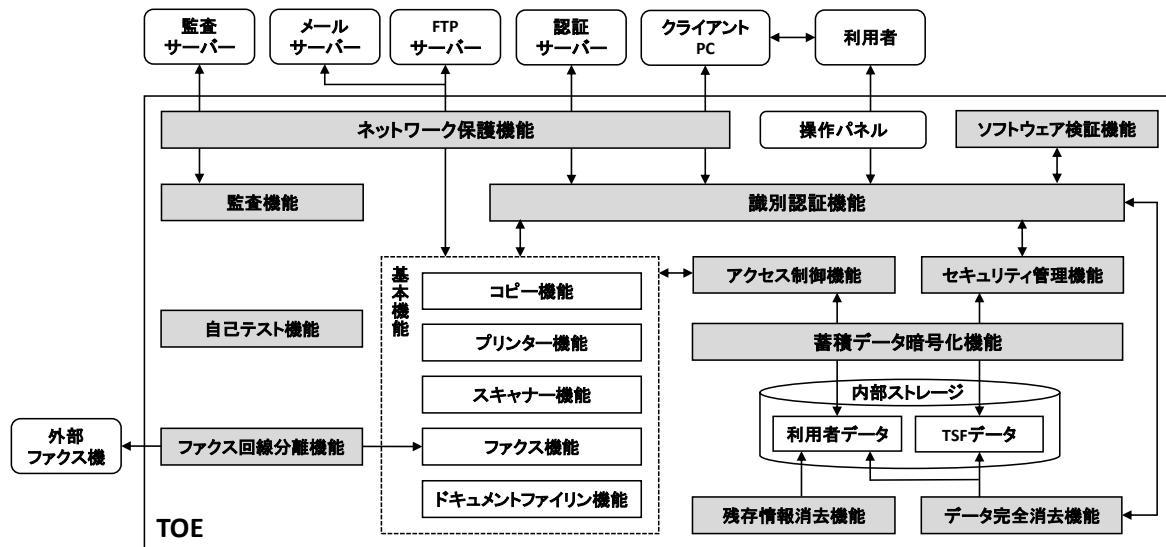
図 5-1 TOE境界
