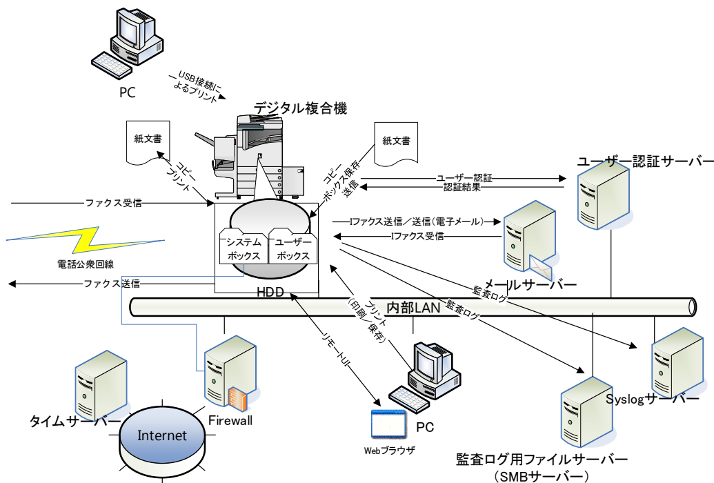
Figure 1 デジタル複合機< Canon imageRUNNER ADVANCE 6500 III Series ファクス付き>の想定設置使用環境
