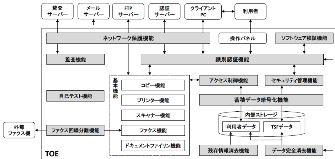
図 5-1 TOE境界
