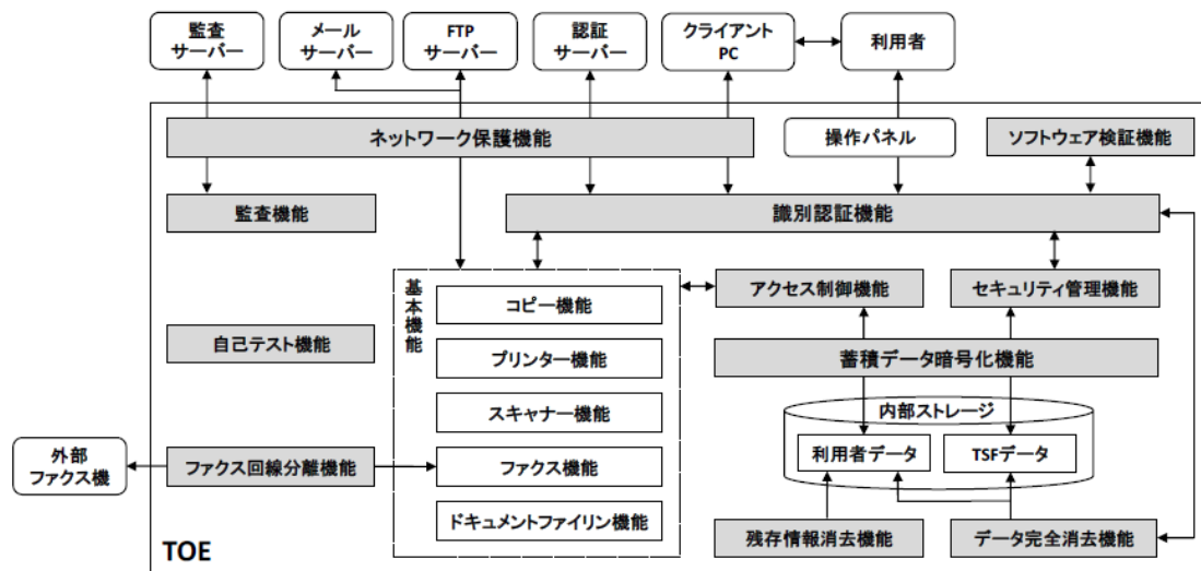
図 5-1 TOE境界
