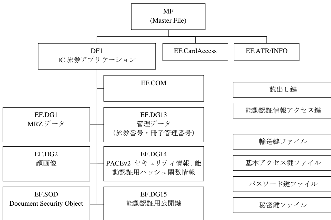
図 1-1 旅券冊子用ICのファイル構成
