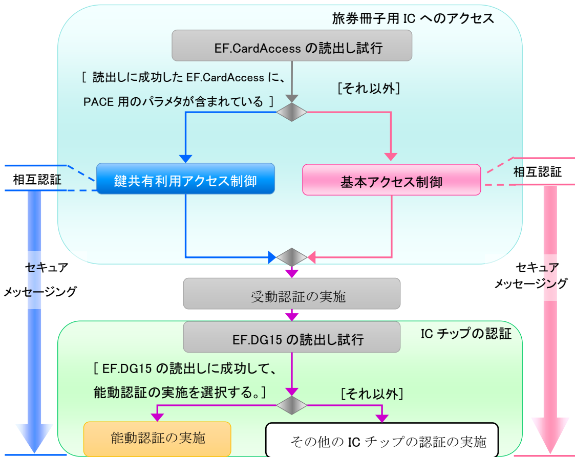
図 1-2 端末装置が旅券冊子用 IC にアクセスする手順
