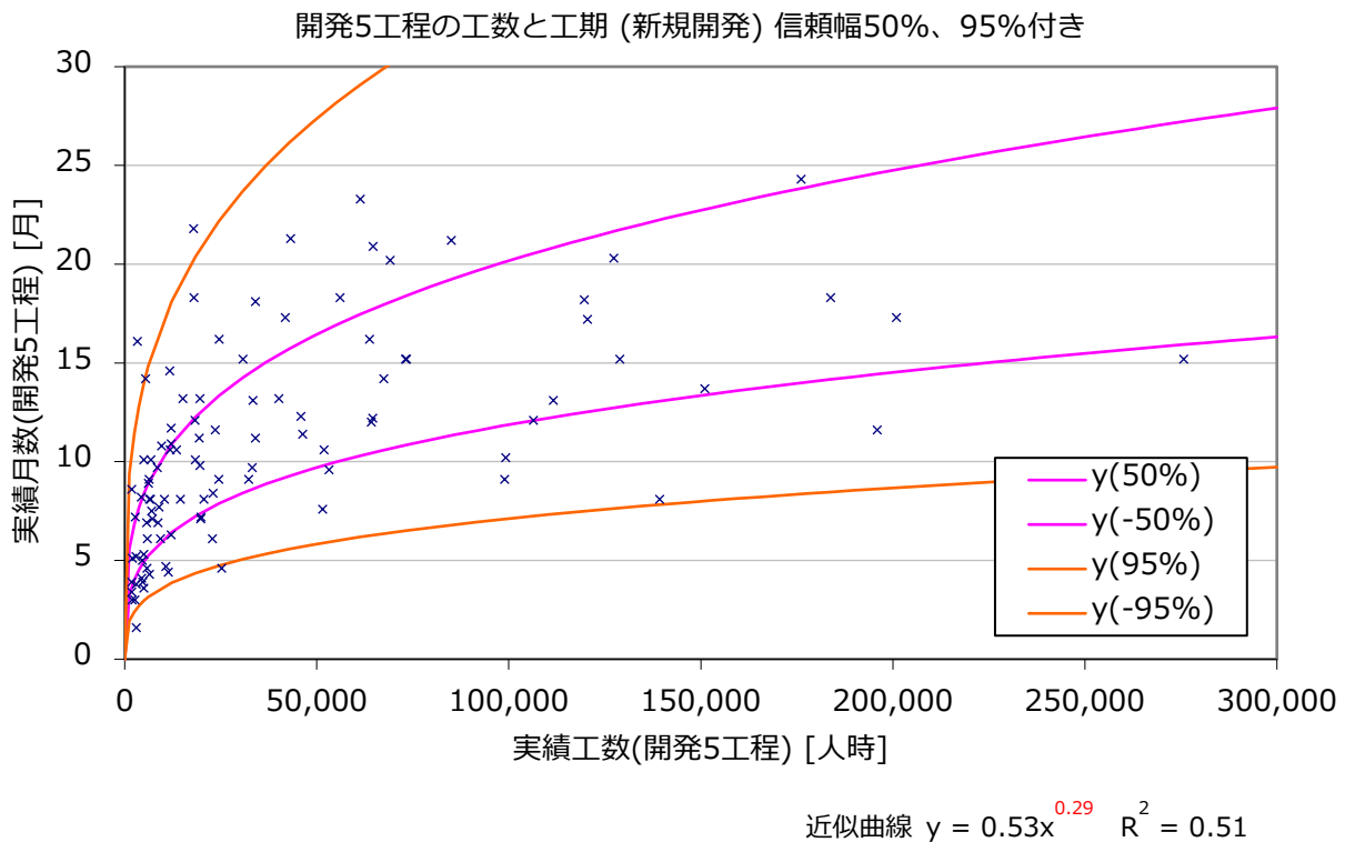
図 A3-3-2 開発 5 工程の工数と工期(新規開発)(信頼区間 50%、95%付き)
