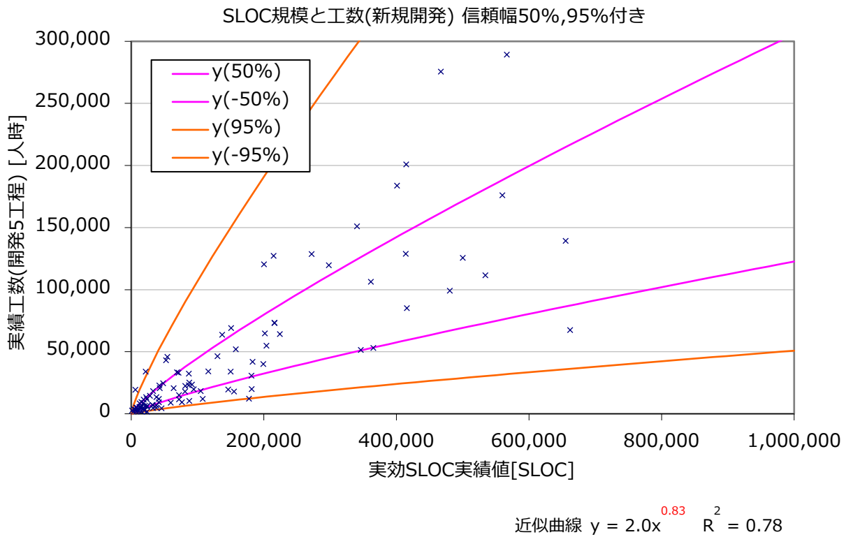
図 A1-1-2 SLOC 規模と工数(新規開発)
