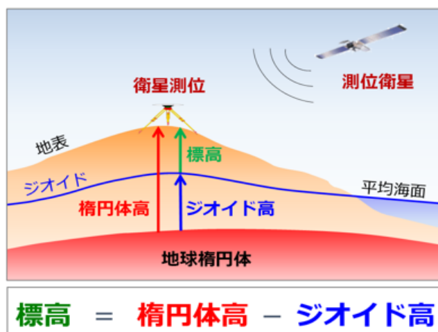
図 2-3 楕円体高、ジオイド高、標高の関係
