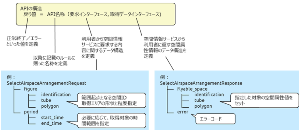
図 3-3 API の概略
