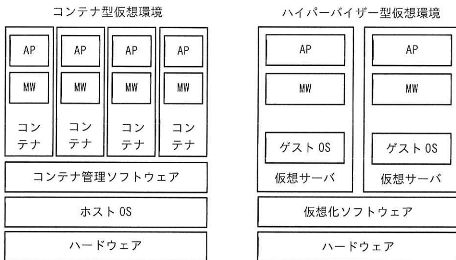
図 1 コンテナ型仮想環境とハイパーバイザー型仮想環境の構成例
