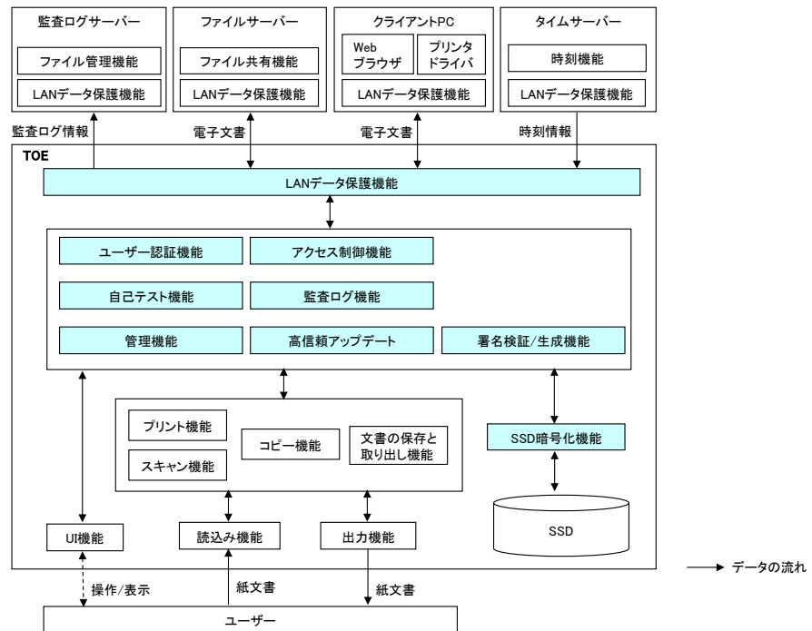
図 5-1 TOE の構成
