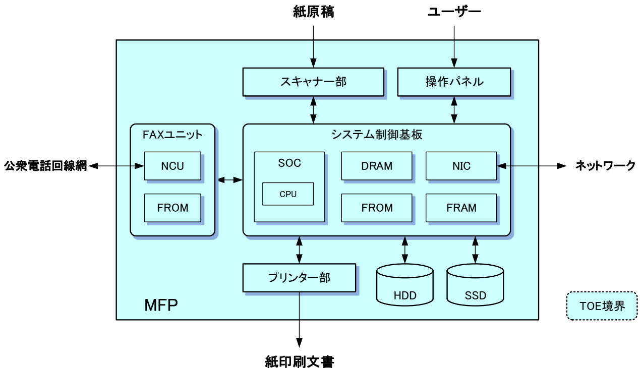
図 2 物理的境界
