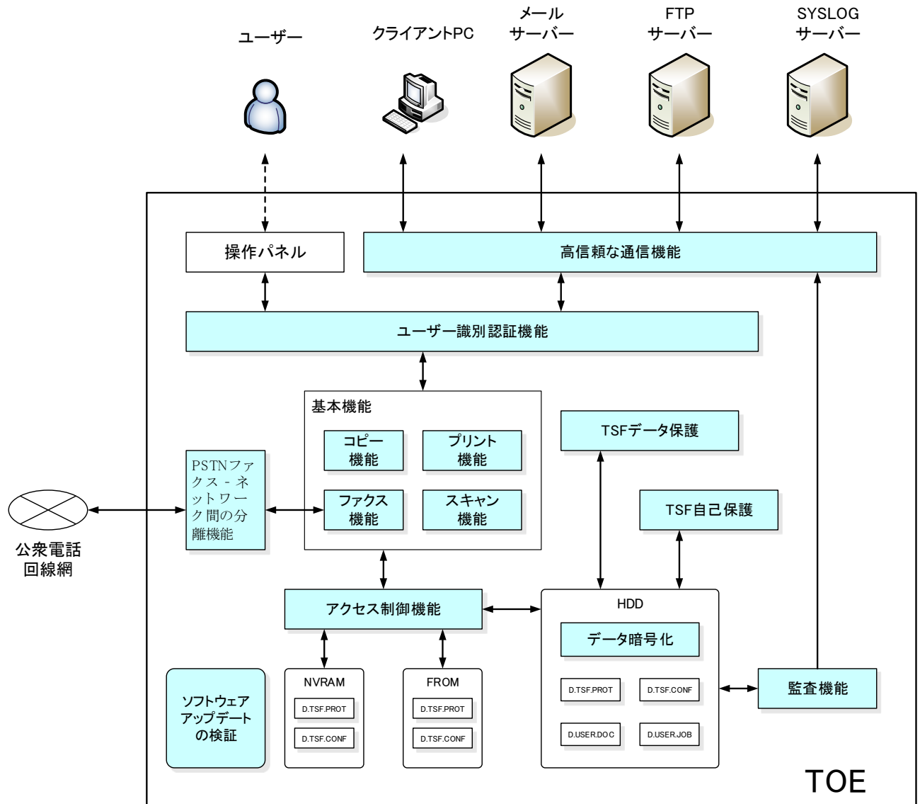
図5-1 TOE 境界
