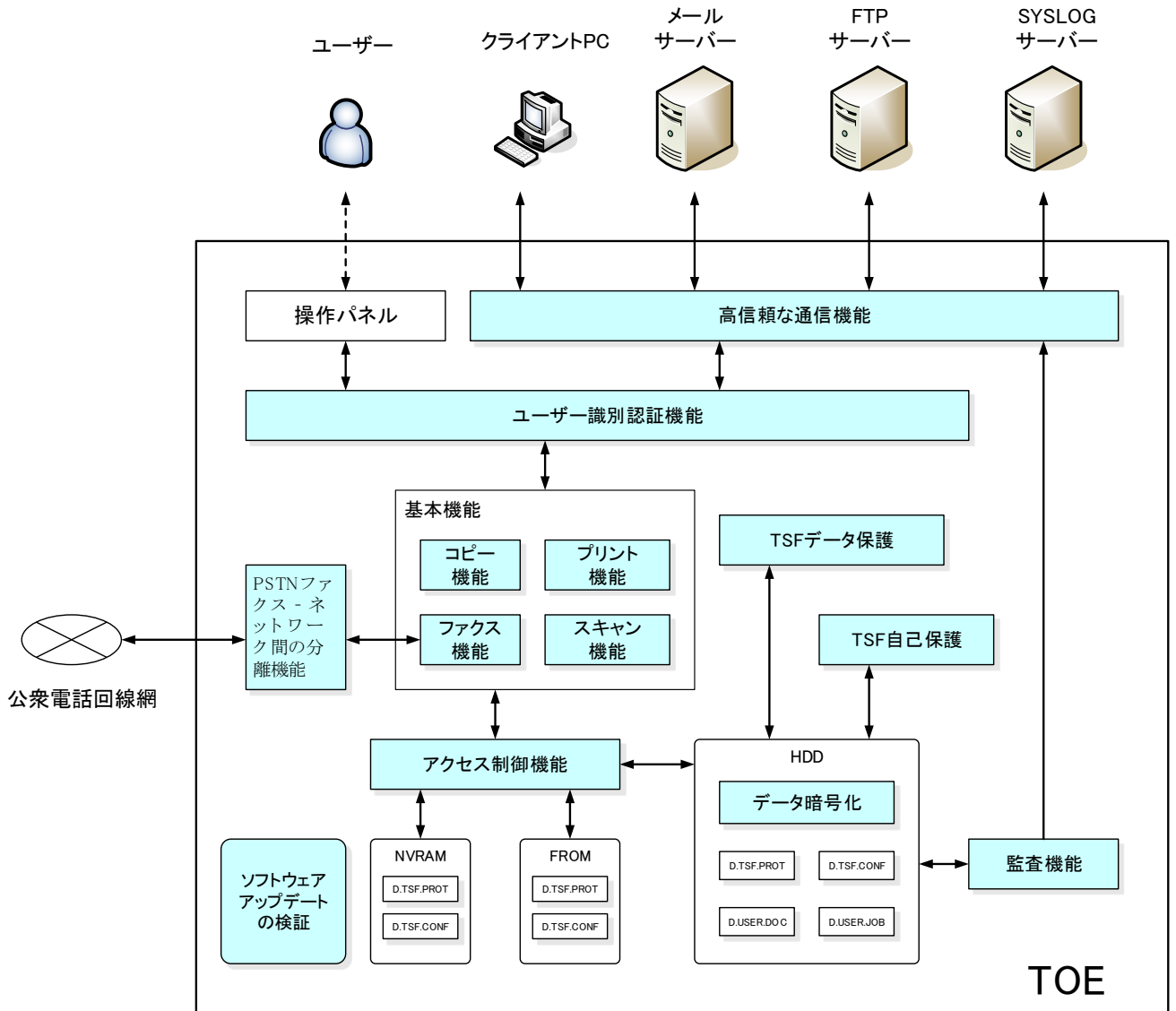
図5-1 TOE 境界
