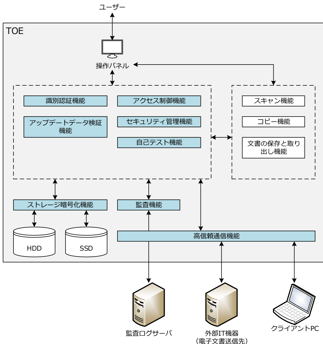
図 5-1 TOE の構成
