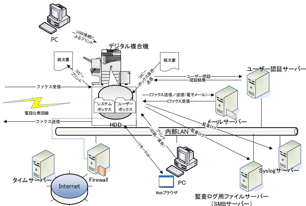
Figure 1 デジタル複合機< Canon imageRUNNER ADVANCE DX 8700 Series ファクス付き >の運用環境
