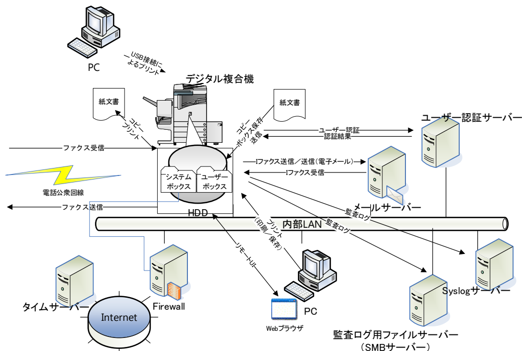
Figure 1 デジタル複合機< Canon imageRUNNER ADVANCE DX C7700 Series ファクス付き >の運用環境
