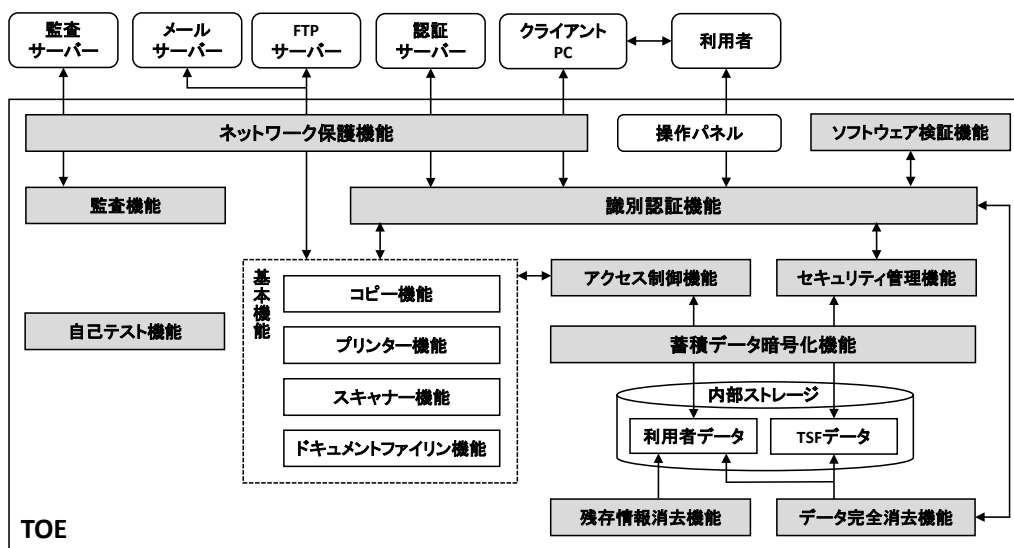
Figure 3: TOE の論理的構成
