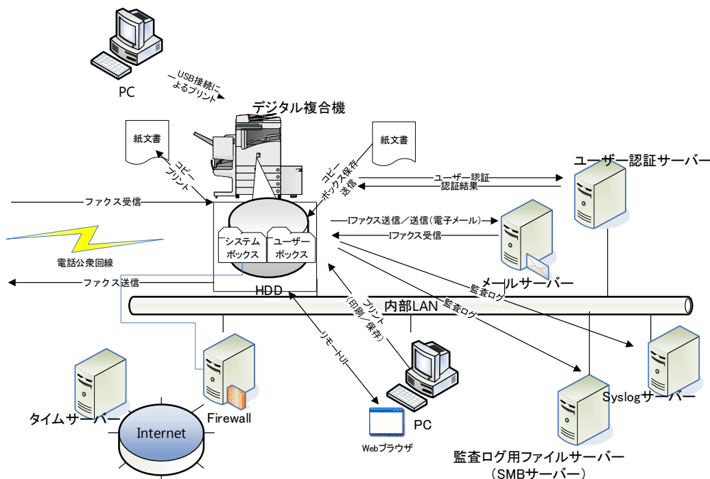
Figure 1 デジタル複合機< Canon imageRUNNER ADVANCE DX C357/C257 Series ファクス付き>の運用環境
