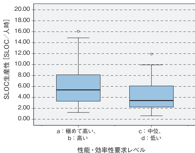
図表 8-4-10 ● 性能・効率性の要求レベル別の SLOC 生産性（新規開発）箱ひげ図
