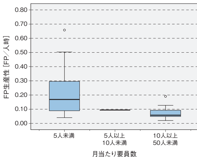
図表 8-4-5 ● 月あたりの要員数別のFP生産性（新規開発）箱ひげ図
