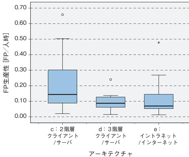
図表 8-4-3 ● アーキテクチャ別のFP生産性（新規開発）箱ひげ図
