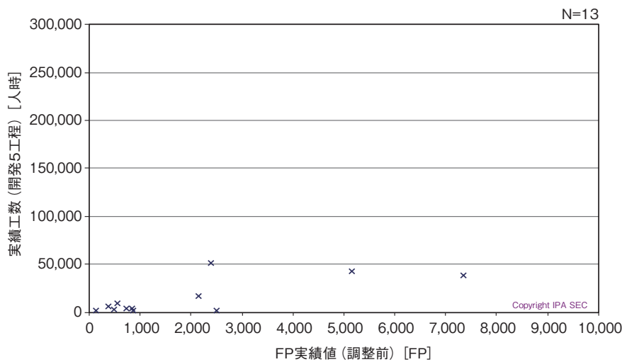
図表 6-3-4 ● FP 規模と工数（新規開発）
