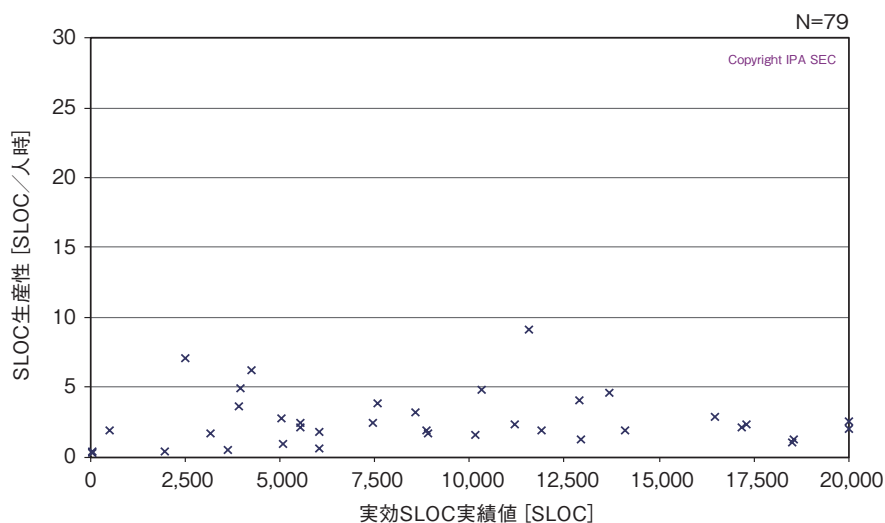
図表 8-3-6 ● SLOC 規模と SLOC 生産性 (改良開発) 拡大図 (SLOC 規模 &lt; 20K)
