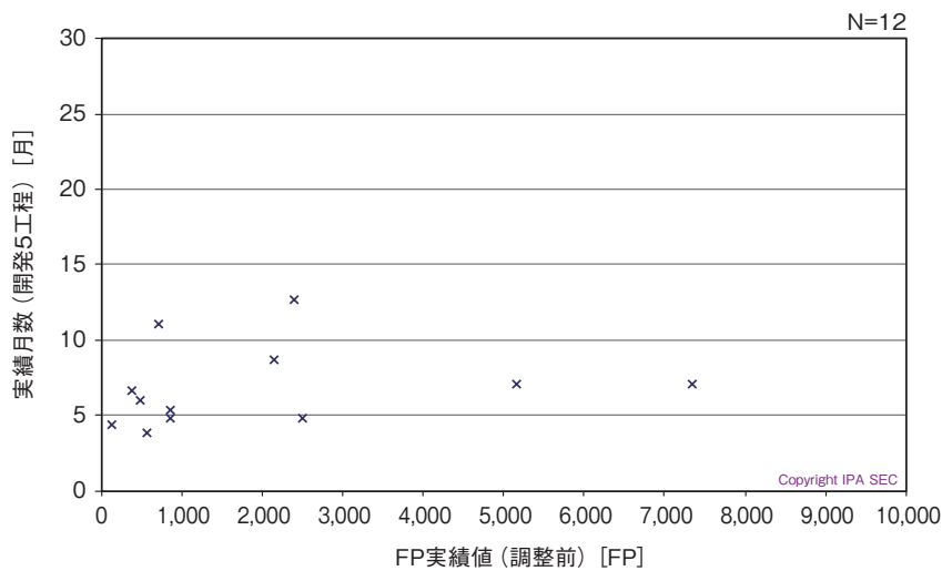
図表 6-5-3 ● FP 規模と工期（新規開発）
