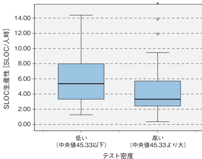
図表 8-4-14 ● テスト密度別の SLOC 生産性（新規開発）箱ひげ図
