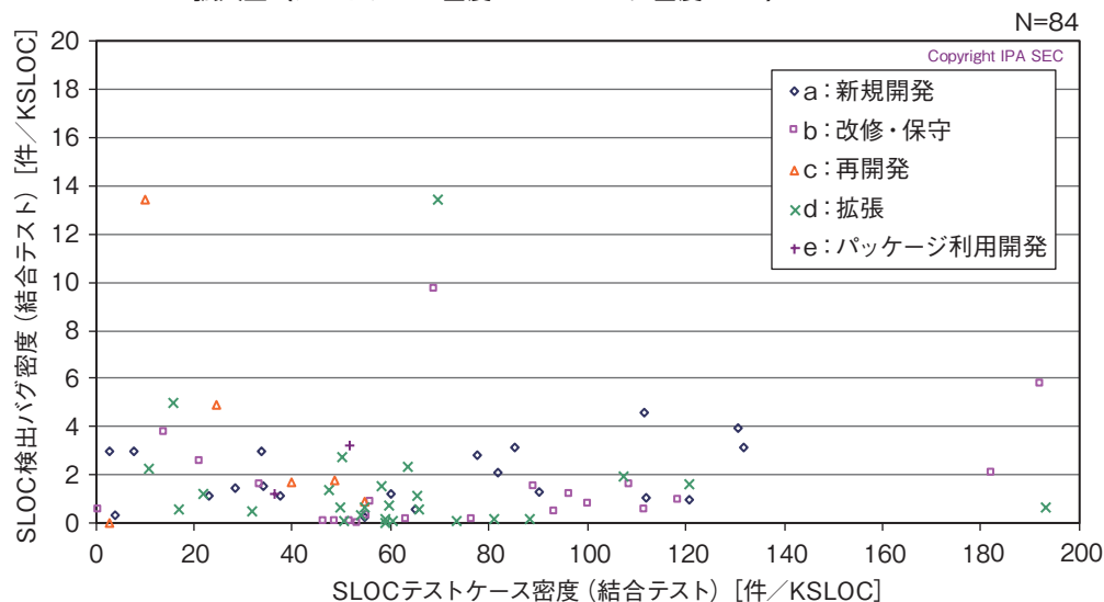
図表 7-5-22 ● SLOC 規模あたりのテストケース数と SLOC 規模あたりの検出バグ現象数 (結合テスト、全開発種別) 拡大図 (テストケース密度 \leq 200 & バグ密度 \leq 20 )
