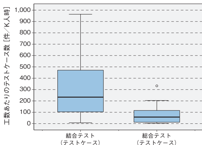
図表 7-5-51 ● 工数あたりのテストケース数（新規開発）箱ひげ図
