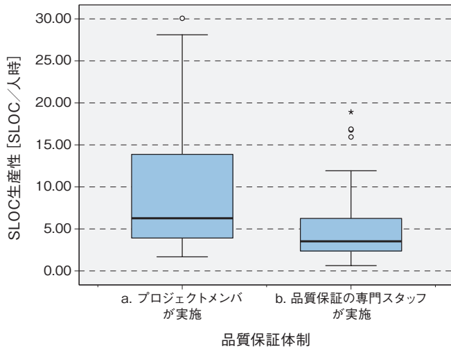
図表 8-4-12 ● 品質保証体制別の SLOC 生産性（新規開発）箱ひげ図
