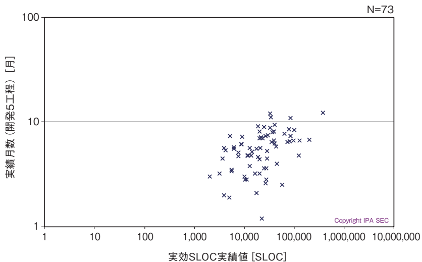
図表 6-6-6 ● SLOC 規模と工期 (改良開発) 対数表示
