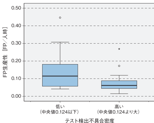
図表 8-4-7 ● テスト検出不具合密度別の FP 生産性 (新規開発) 箱ひげ図
