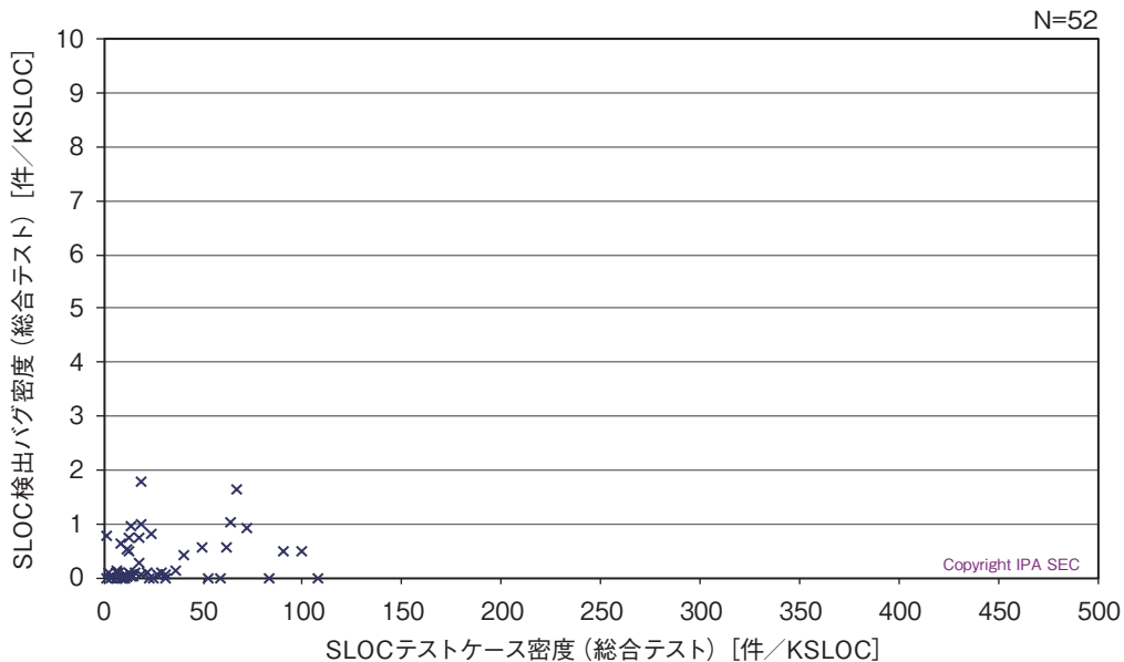
図表 7-5-35 ● SLOC 規模あたりのテストケース数と SLOC 規模あたりの検出バグ現象数 (総合テスト (ベンダ確認)、改良開発)
