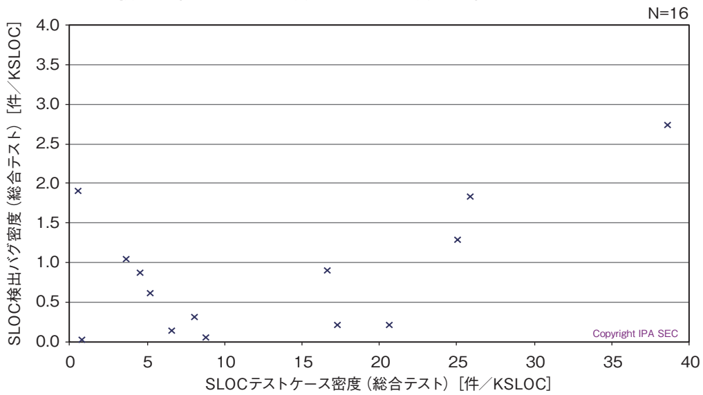
図表 7-5-30 ● SLOC 規模あたりのテストケース数と SLOC 規模あたりの検出バグ現象数 (総合テスト (ベンダ確認)、新規開発) 拡大図 (テストケース密度 ≤ 40 & バグ密度 ≤ 4.0)
