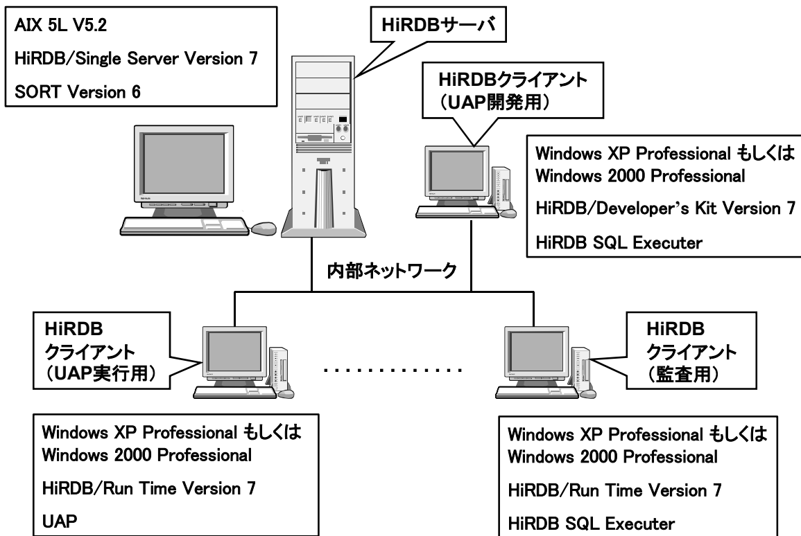
図 2-1 : HiRDB / Single Server Version 7 を含むシステム構成
