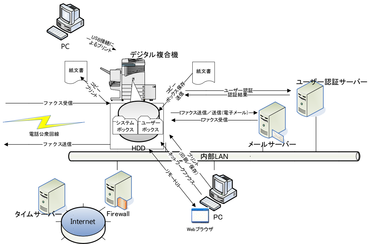
Figure 1 デジタル複合機< Canon imageRUNNER ADVANCE C355/C255 Series >の想定設置使用環境
