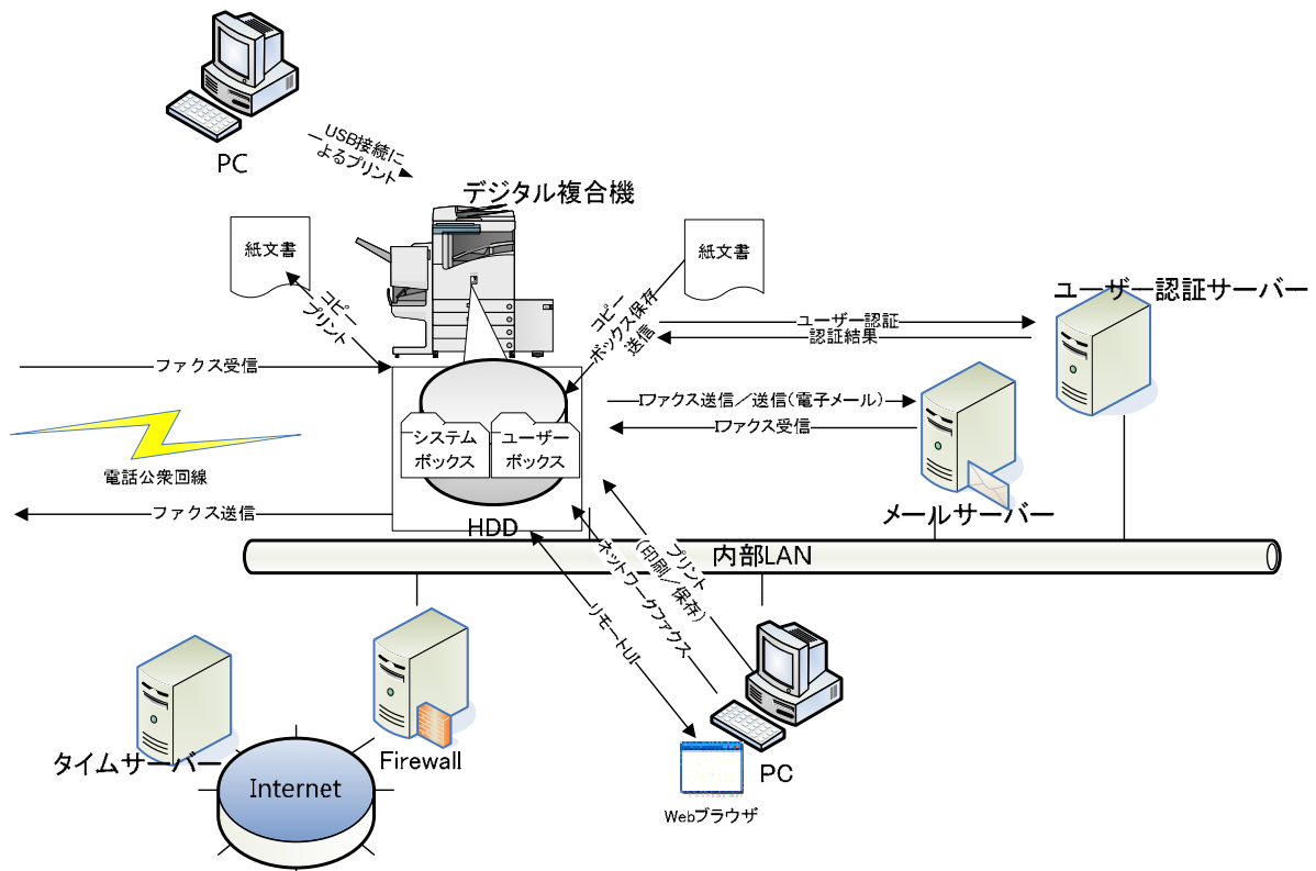
Figure 1 デジタル複合機< Canon imageRUNNER ADVANCE 4200 Series >の想定設置使用環境
