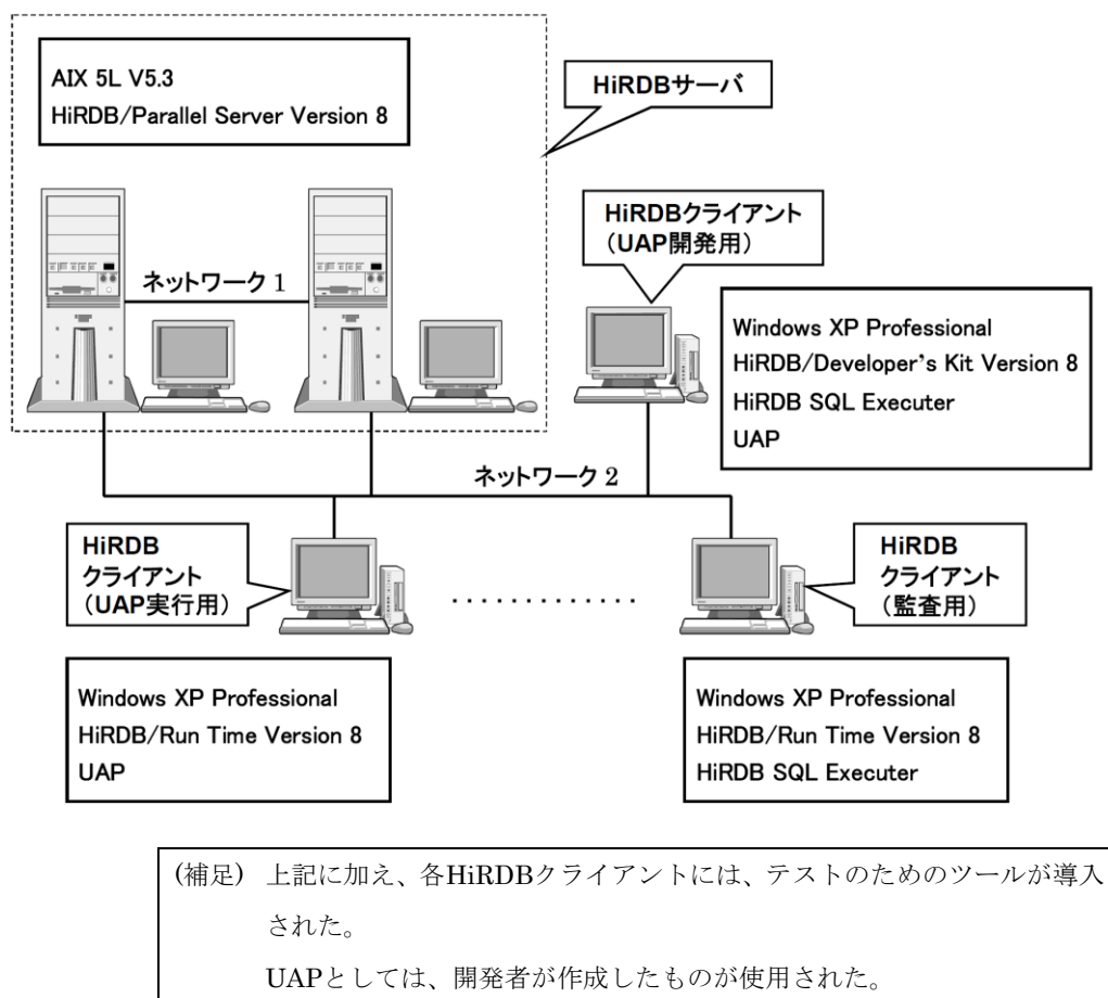
図2-1 開発者テストの構成図
