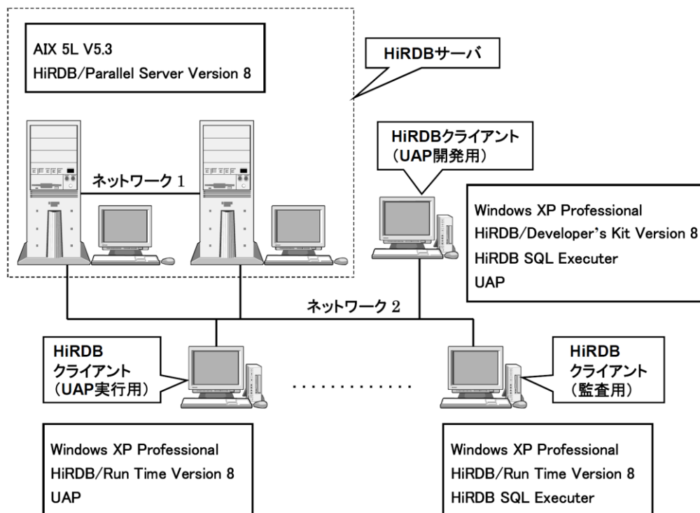
図1-3 TOEの動作環境
