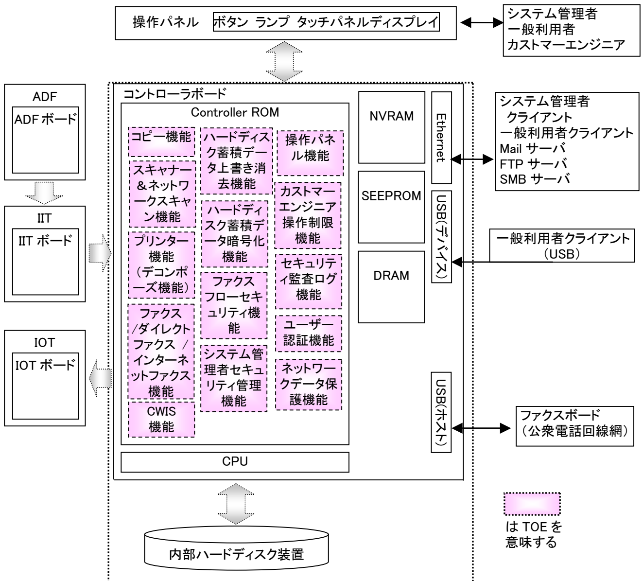
図 4 MFP 内の各ユニットと TOE の物理的範囲
