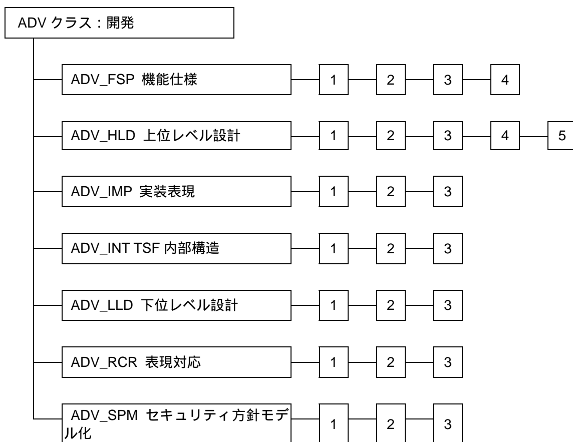
図 10.1 - 開発クラスのコンポーネント構成
