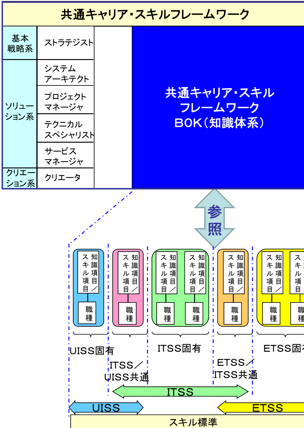
【図1】 知識体系 (BOK) とスキル標準(レベル1～4) の構造
