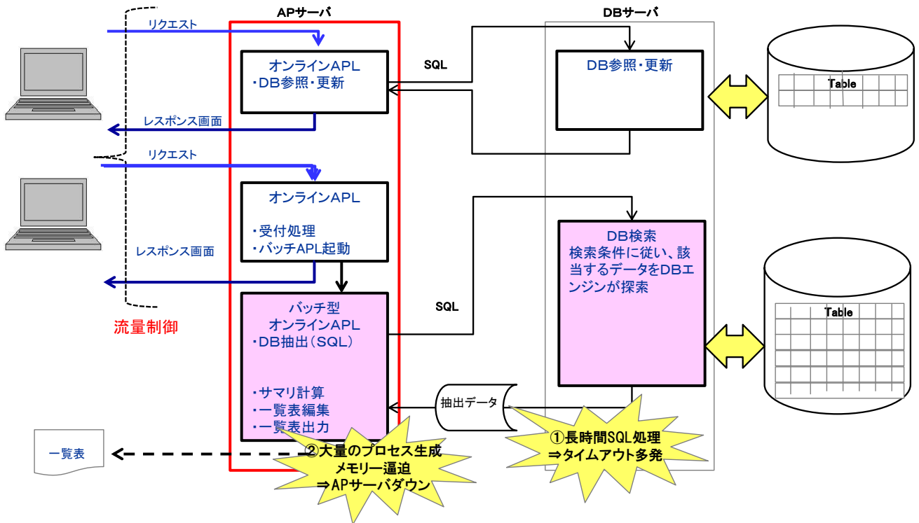
図 2. 5 - 1 本システムの概要と障害の流れ
