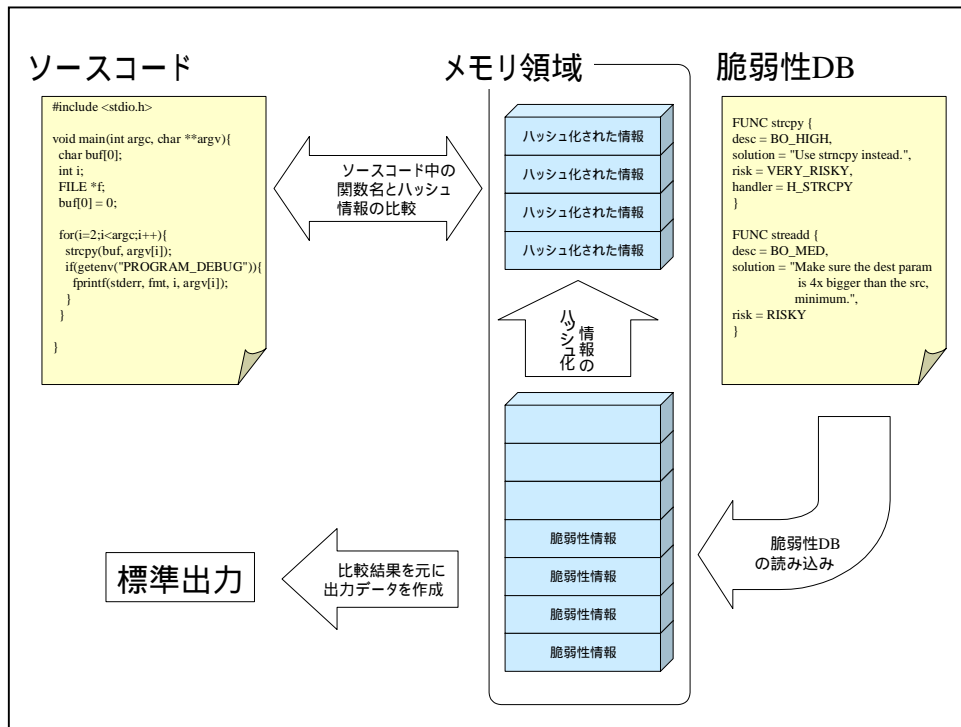
図4. ITS4 の動作
