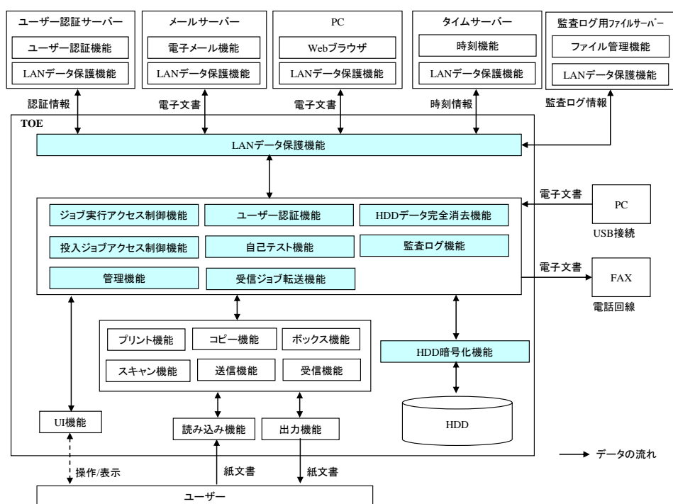
図5-1 TOE境界
