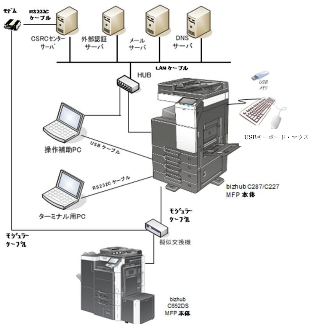
図7-1 開発者テストの構成図
