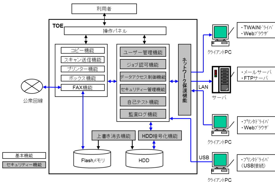
図 5-1 TOE の構成
